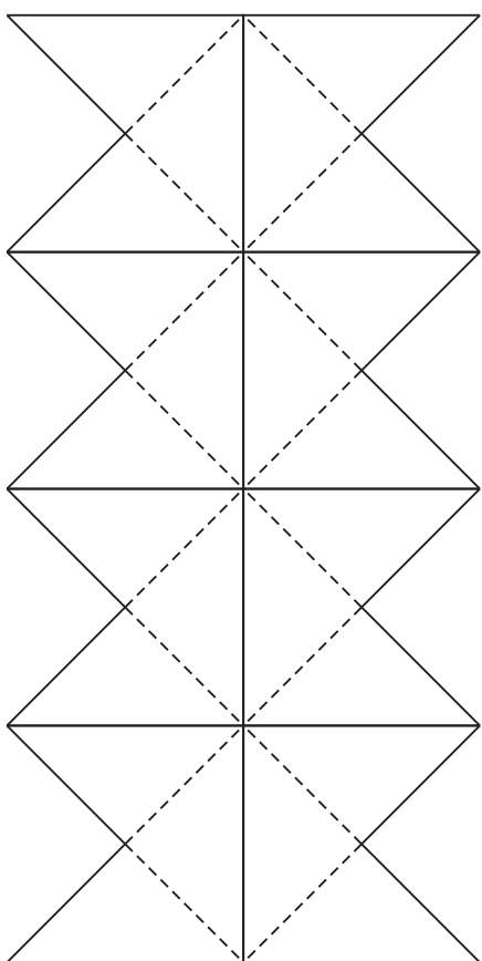
šestistěn
