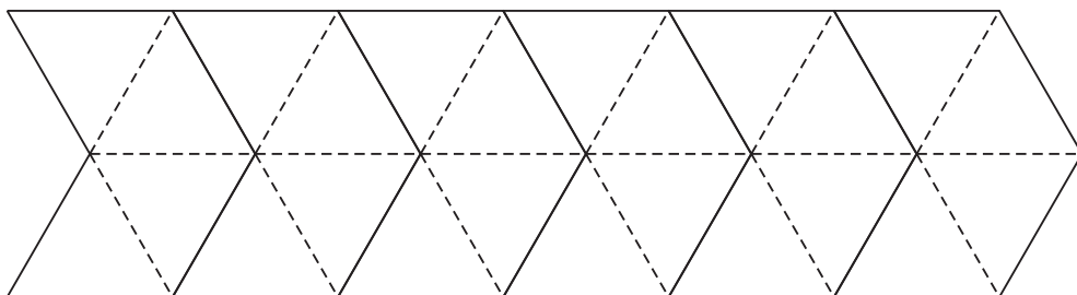
osmistěn
